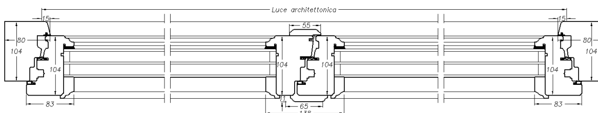
Sezione B-B'
