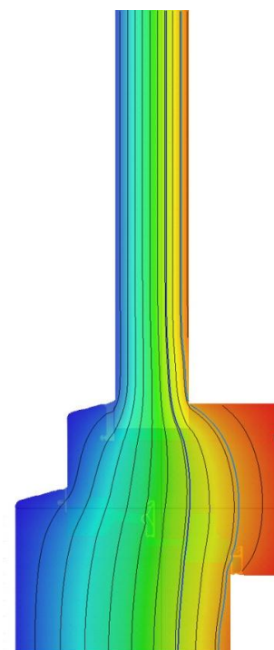
Isoterme
